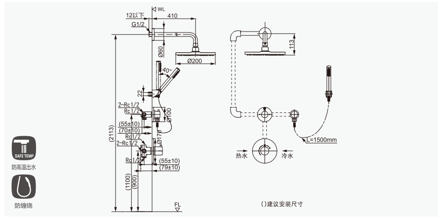
①入墙壁式花洒 FFIX9SMA-245500BC0 ②入墙式操控本体(附阀芯) FFIX4921-604500BC0 入墙式操控面板 FF1-CN522X70066999 ③入墙式赛沐操控本体(附阀芯) FFIXBT21-604500BC0 入墙式赛沐操控面板 FF1-CN522X70066799 ④墙面连接器 FFIXMAC0-283500BC0 ⑤手持花洒 FFIX9HBF-13C500BC0
