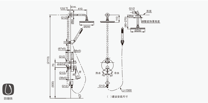
①入墙壁式花洒 FFIX9SMA-245500BC0 ②入墙式操控本体(附阀芯) FFIXBE21-604500BC0 入墙式操控面板 FFI1-CN522X70067199 ③墙面连接器 FFIX97MA-025500BC0 ④手持花洒 FFIX9HBF-13C500BC0 ⑤顶置式花洒 FFIX9SMA-307500BC0
