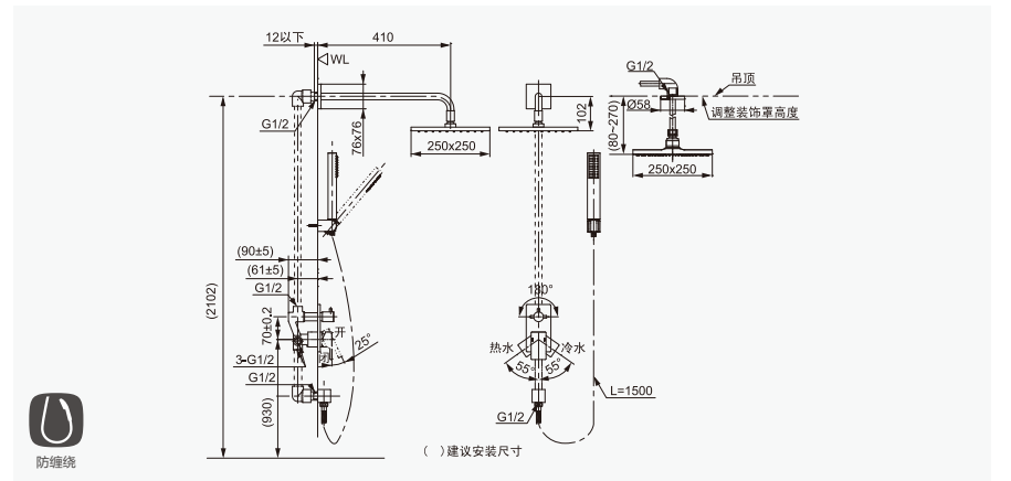
① 入墙壁式花洒 FFIX9SMA-306500BC0 ② 入墙式操控本体 (附阀芯) FFIXBJ21-604500BC0 入墙式操控面板 FF1-CN522X70066899 ③ 墙面连接器 FFIX97MA-075500BC0 ④ 手持花洒 FFIX9HBF-14C500BC0
