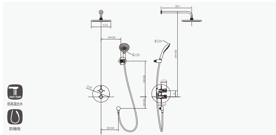
· 恒温二路出水暗藏花洒(黑色) · 恒温阀芯 · 预埋阀芯 FF1-CN522X70079599 · 手持花洒按键切换 · 其他 FF1-CN522X70079799 · 手持花洒多种出水模式: 花洒水, 按摩水, 中空水 · 高雅黑色表面
