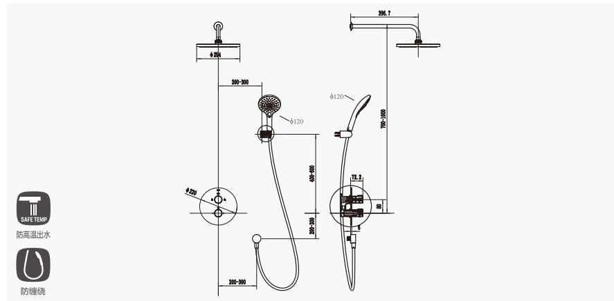
· 恒温二路出水暗藏花洒(银色) · 恒温滤芯 · 预埋滤芯 FF1-CN522X70079299 · 手持花洒按键切换 · 顶洒+支臂 FF1-CN522X70079399 · 手持花洒多种出水模式：花洒水，按摩水，中空水 · 其他 FF1-CN522X70079499 · 优质表面镀层
