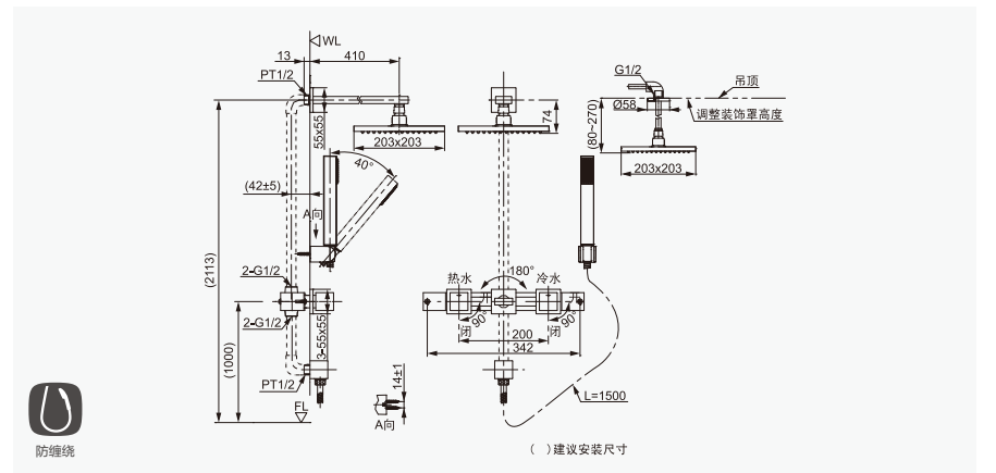
①入墙壁式花洒 FFIX9SMA-275500BC0 ②入墙式操控本体(附阀芯) FFIXBD21-604500BC0 入墙式操控面板 FF1-CN522X70066499 ③墙面连接器 FFIX97MA-075500BC0 ④手持花洒 FFIX9HBF-14C500BC0 ⑤顶置式花洒 FFIX9SMA-310500BC0
