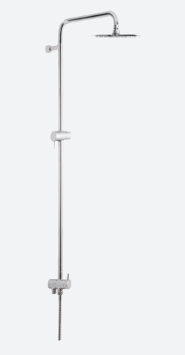
花洒淋浴柱 FFIX9R06-000500BC0
