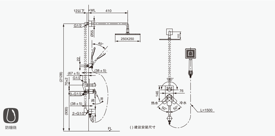
①入墙壁式花洒 FFIX9SMA-306500BC0 ②入墙式操控本体(附阀芯) FFIX97MA-420500BC0 入墙式操控面板 FFIX97MA-430500BC0 ③墙面连接器 FFIX97MA-075500BC0 ④手持花洒 FFIX9HBF-19C500BC0
