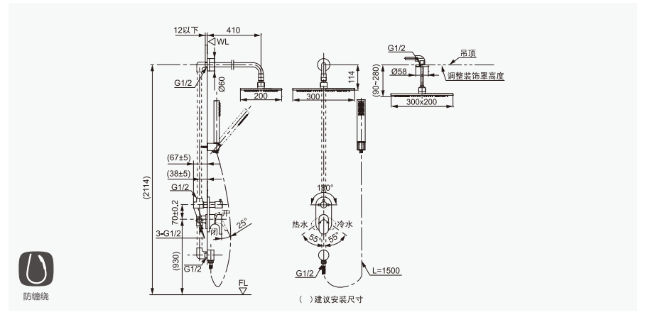
①入墙壁式花洒 FFIX9SMA-305500BC0 ②入墙式操控本体(附调芯) FFIXBH21-604500BC0 入墙式操控面板 FF1-CN522X70066699 ③墙面连接器 FFIX97MA-025500BC0 ④手持花洒 FFIX9HBF-15C500BC0 ⑤置顶式花洒 FFIX9SMA-309500BC0
