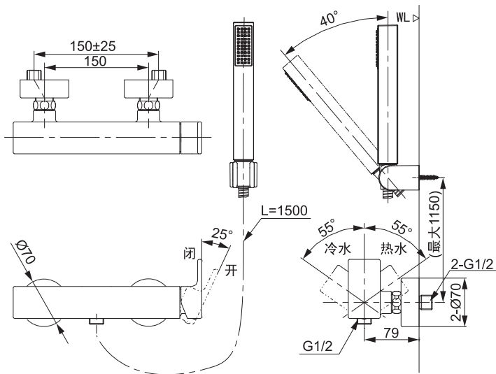
( ) 建议安装尺寸
