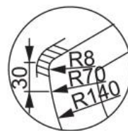
A部详图
