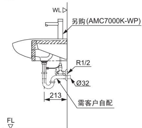
A部详图
