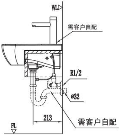
A部详细
