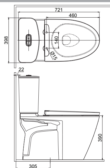
AC-602VN CC060201-6DFC0-AN
